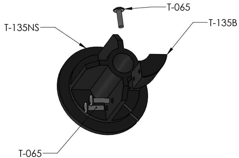
T-BAND4 DETAIL
