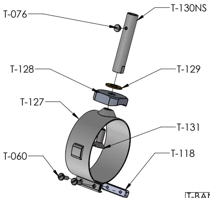
T-BAND2 DETAIL
