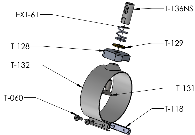
T-BAND4 DETAIL
